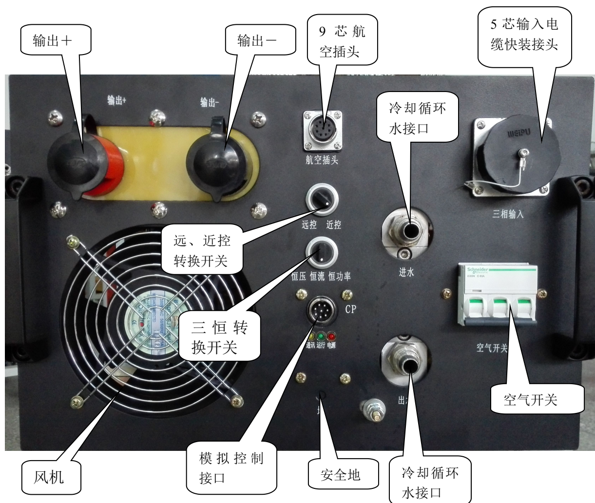
电源后面板示意图 (图二)
